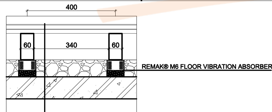
MẶT CẮT PHÒNG TEST ÂM
