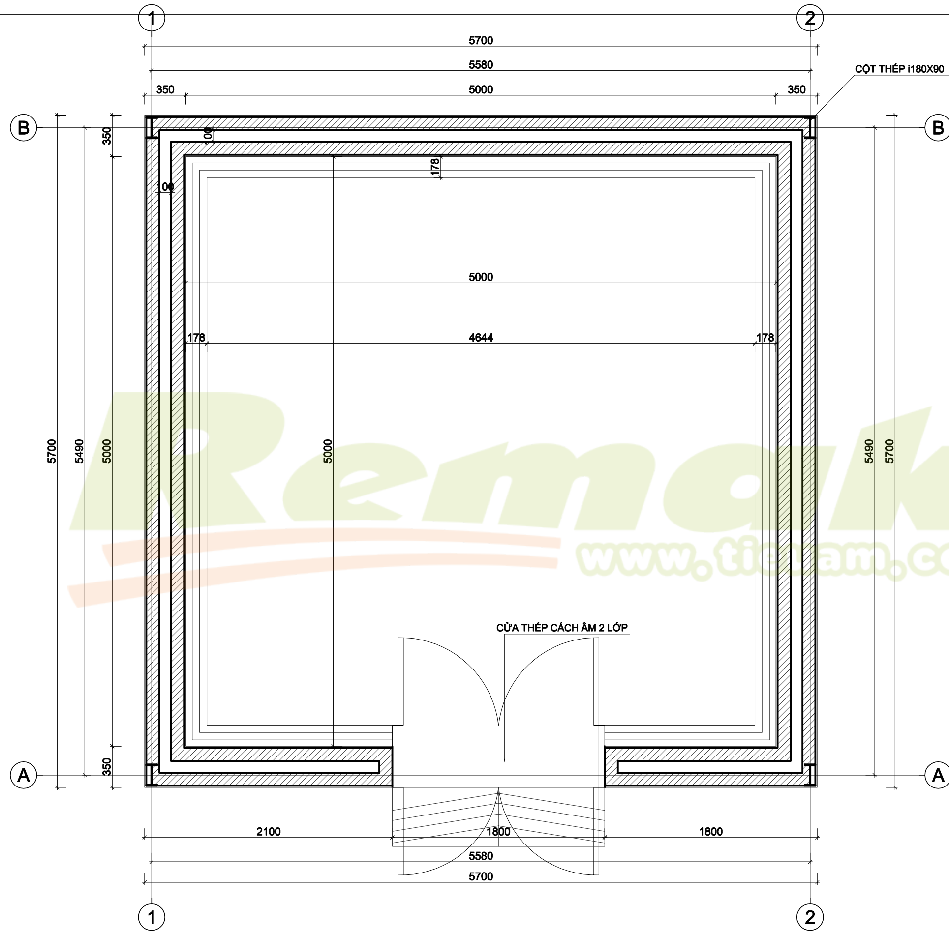
MẶT BẰNG PHÒNG TEST ÂM
