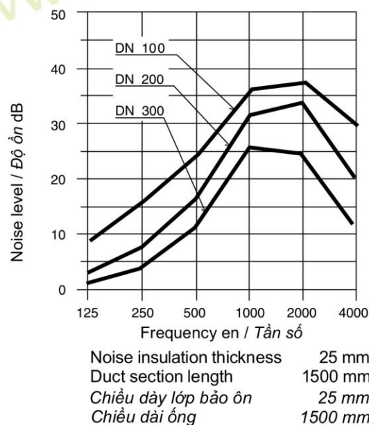
Hình 3: Độ giảm ồn ống gió mềm có bảo ôn
